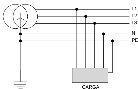
Figura 1 - Esquema TN-S
