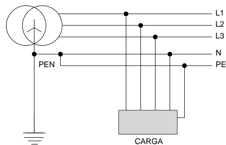
Figura 2 - Esquema TN-C-S
